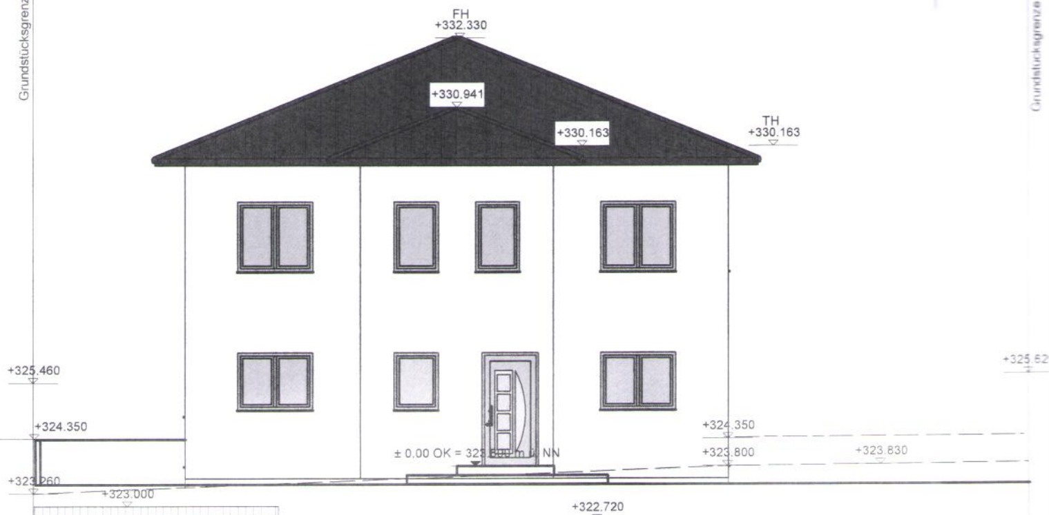
Ansicht Nord
