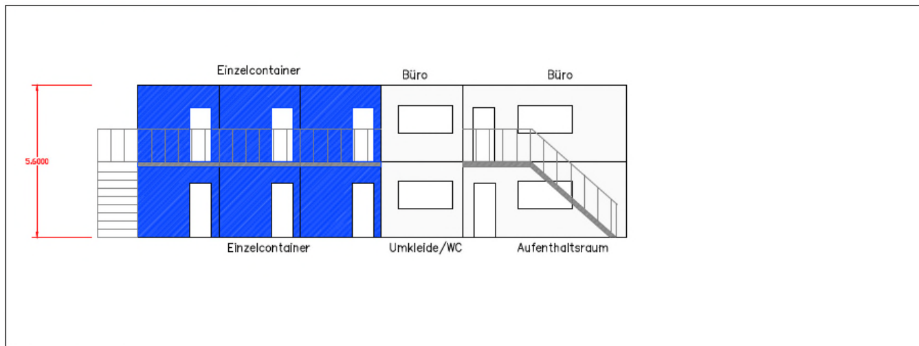
Ansicht 2 M 1:100
