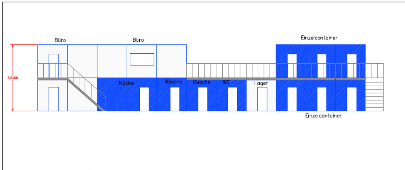
Ansicht 2 M 1:100
