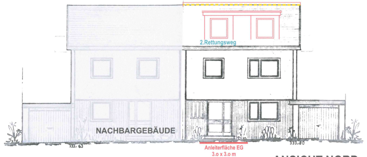
ANSICHT NORD
