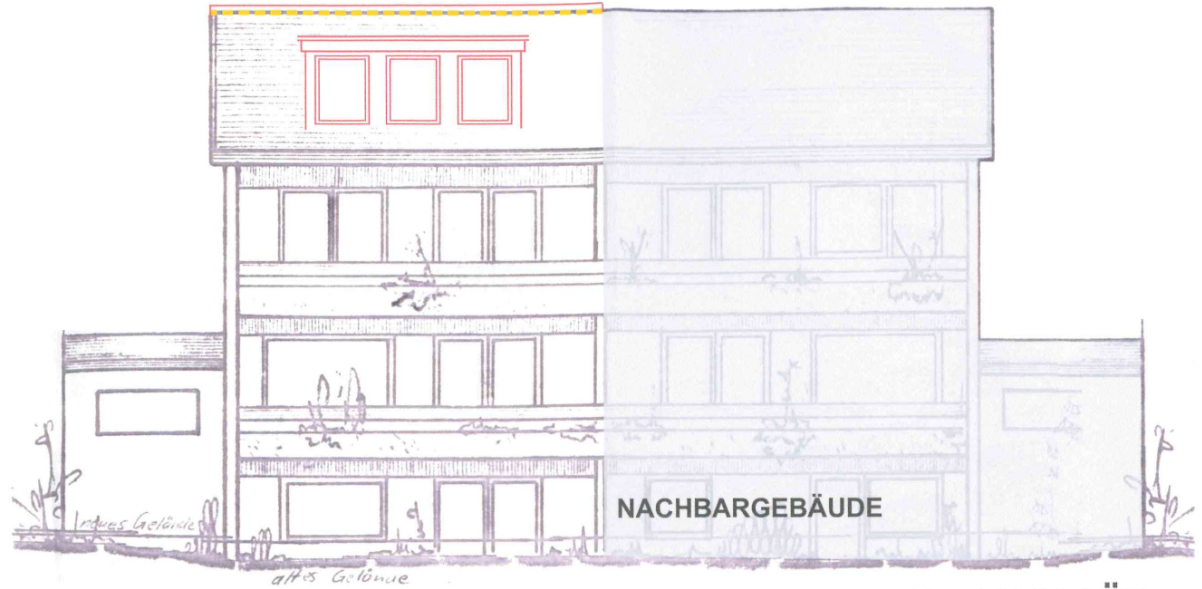
ANSICHT SÜD
