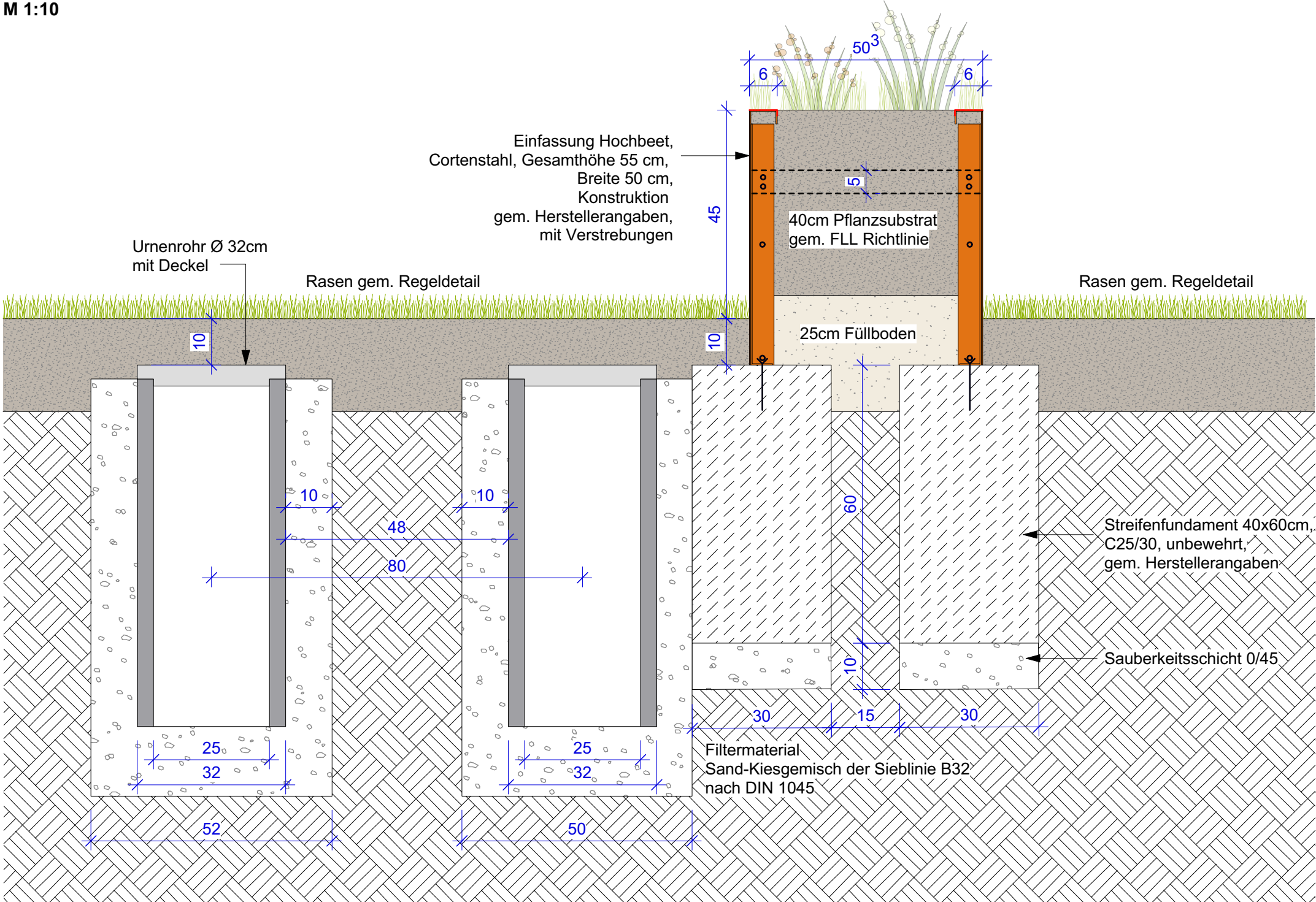
Regeldetail Grabfeld C: Einfassung erhöhte Pflanzbeete mit Urnenrohren M 1:10
