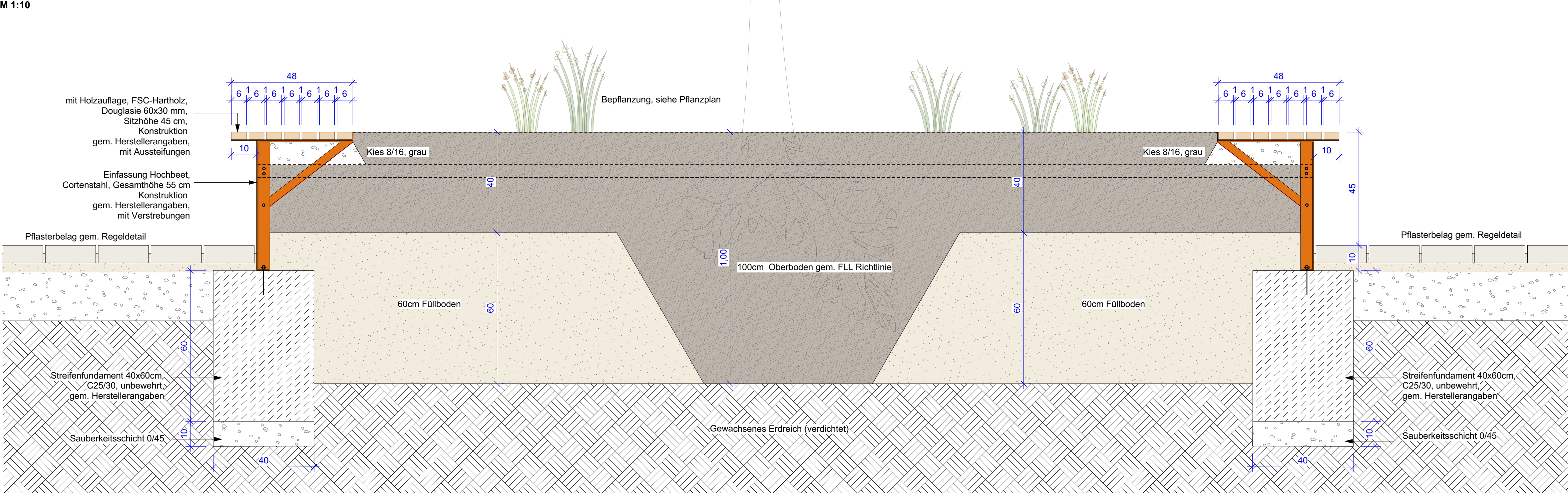
Regeldetail Grabfeld A: Einfassung erhöhtes Pflanzbeet mit Sitzgelegenheiten M 1:10
