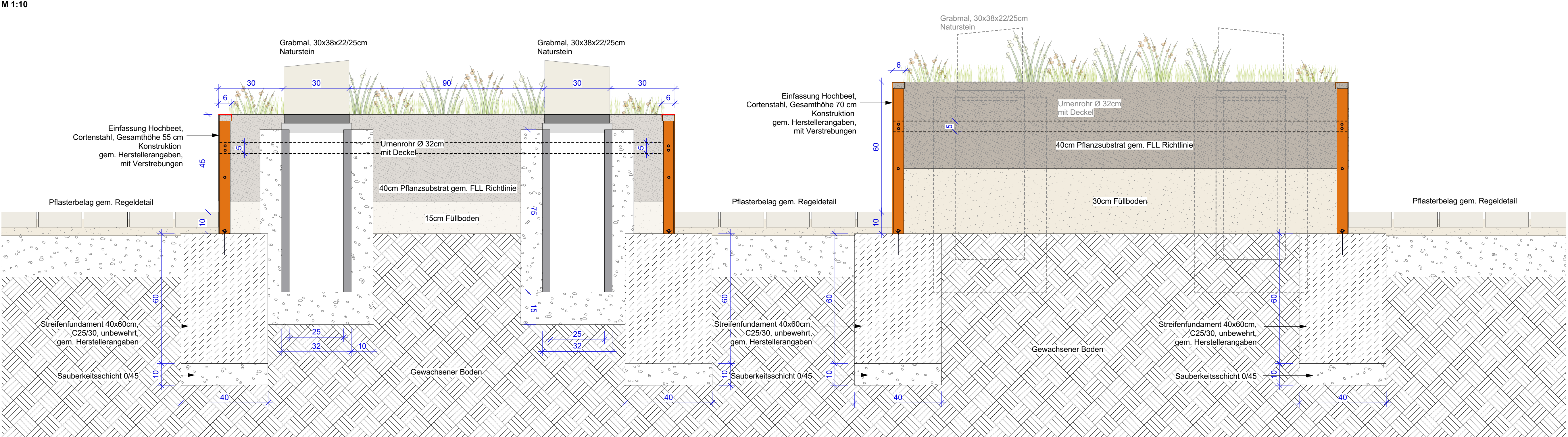
Regeldetail Grabfeld A: Einfassung erhöhte Pflanzbeete mit Urnenrohren M 1:10
