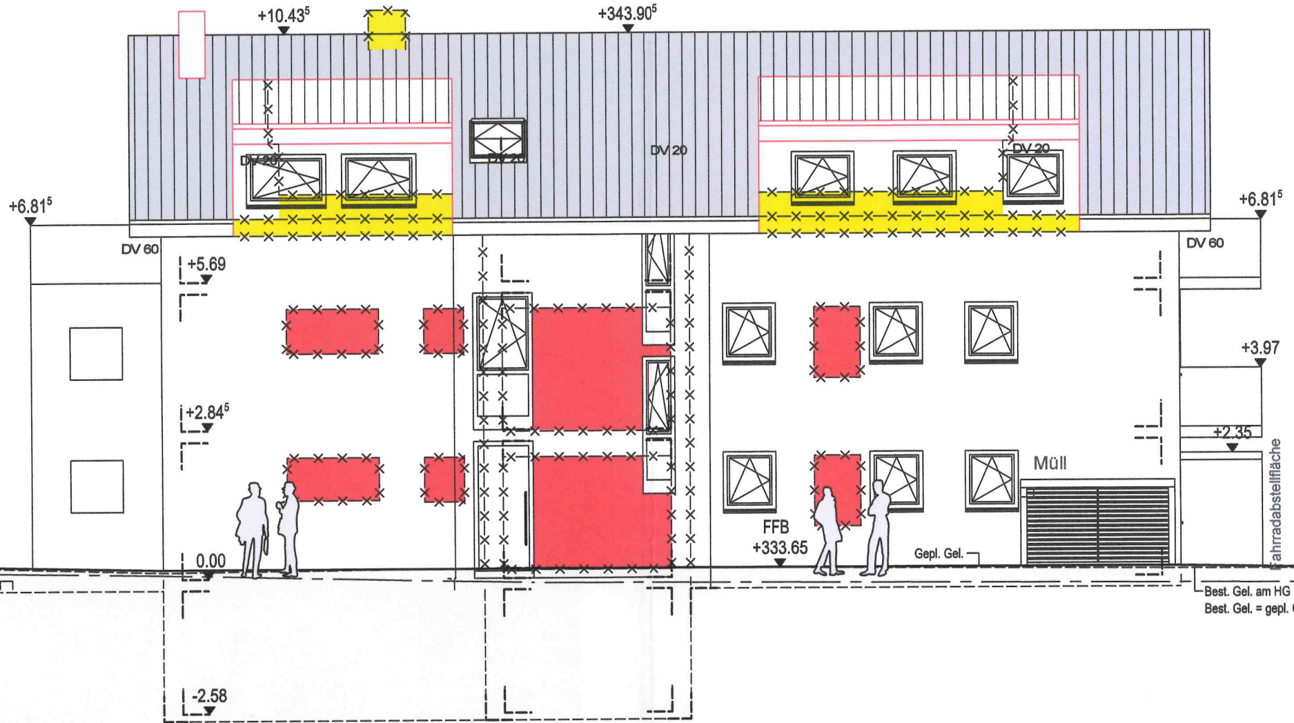
Ansicht Nord
