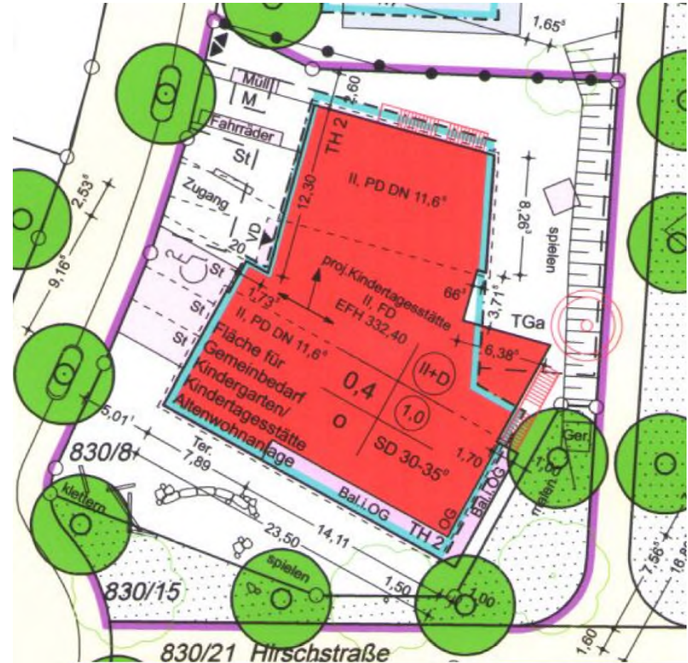
Auszug aus dem Lageplan (04.11.2020) zum Bauantrag für den „Neubau einer Kindertagesstätte“
