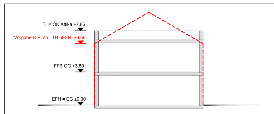
Systemschnitt Gebäudehöhen
