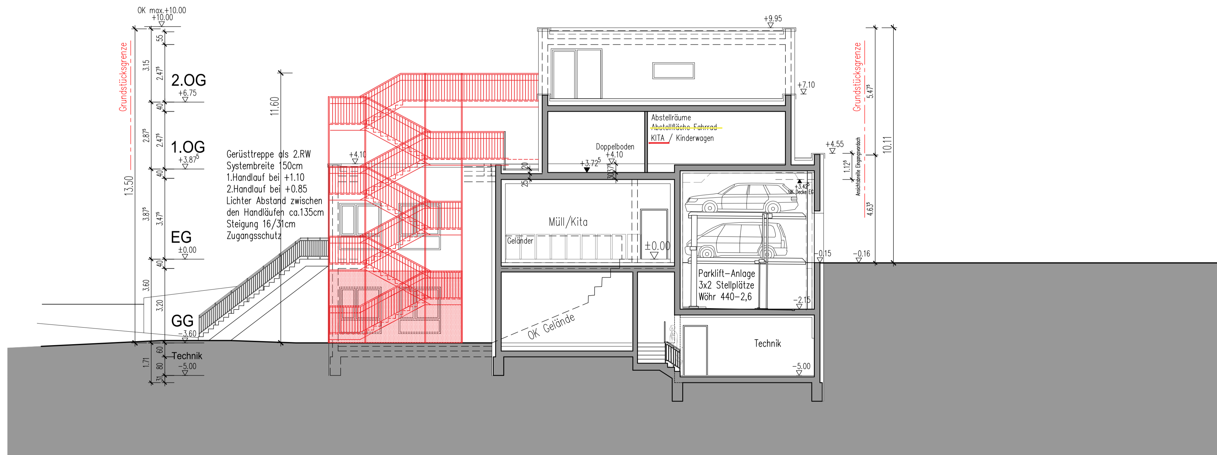
Querschnitt
