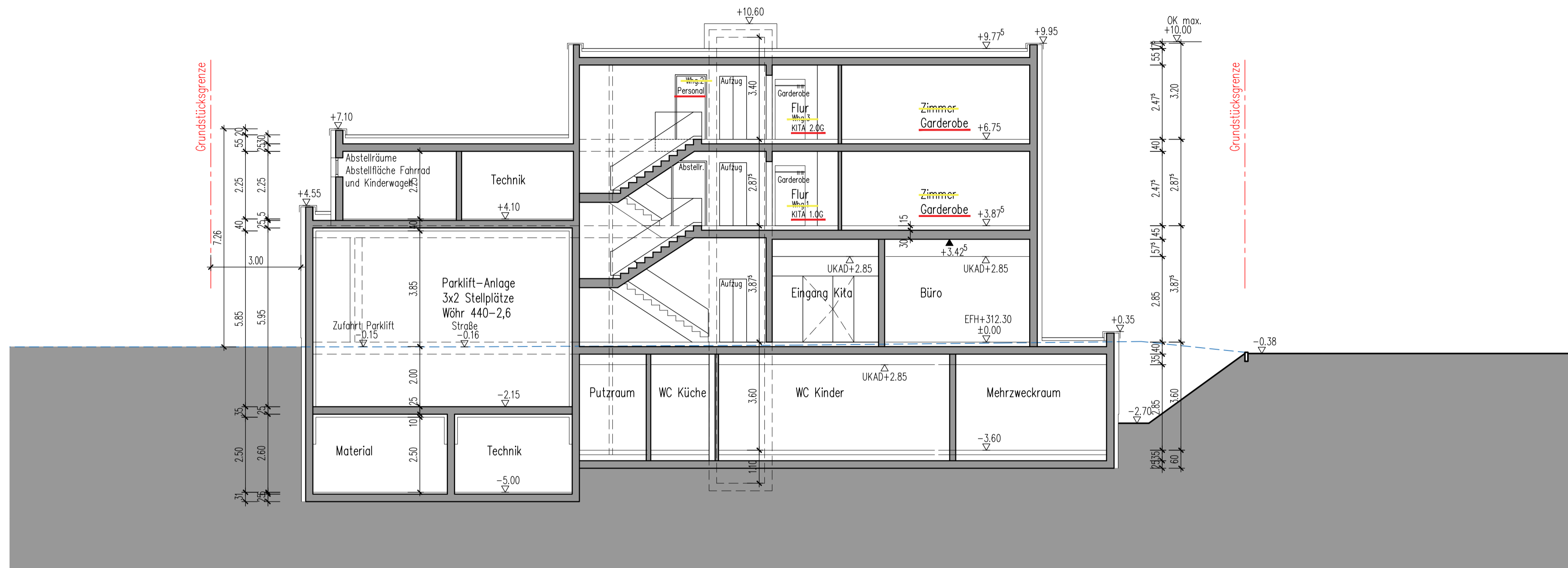
Längsschnitt
