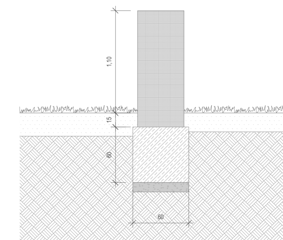
Schnitt quer Helukabelschriftzug M 1:25
